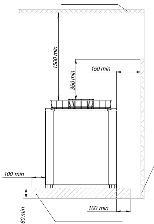
Рисунок-2. Установка электронагревательного устройства
